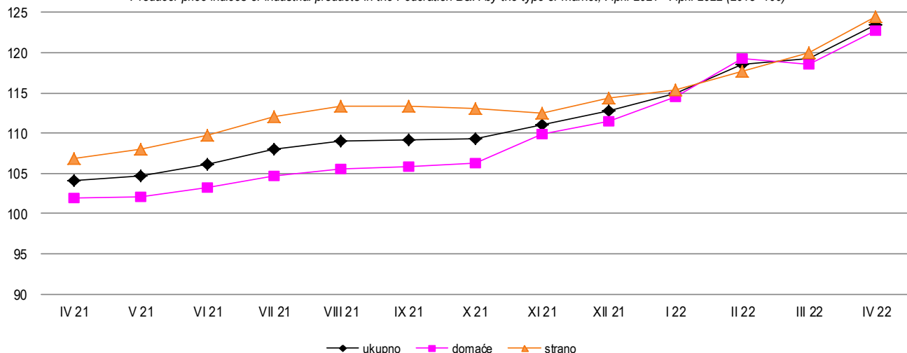
Grafik 1. Indeksi cijena proizvođača industrijskih proizvoda u F BiH po vrsti tržišta, april/travanj 2021 - april/travanj 2022 (2015=100)
